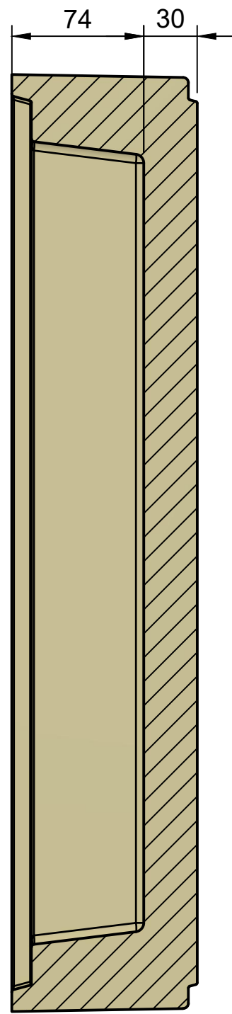
A-A (1:3)
